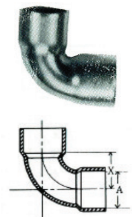
銅エルボ CuEA
