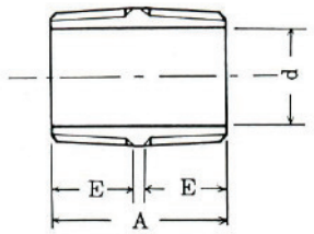
青銅製 (BC-6)
