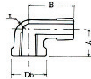
黄銅鍛造製縁付型(C3771)
