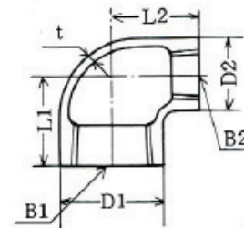
青銅 鑄造平型(BC-6)
