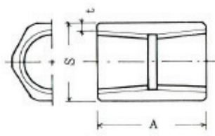
黄銅製 (C3604)
