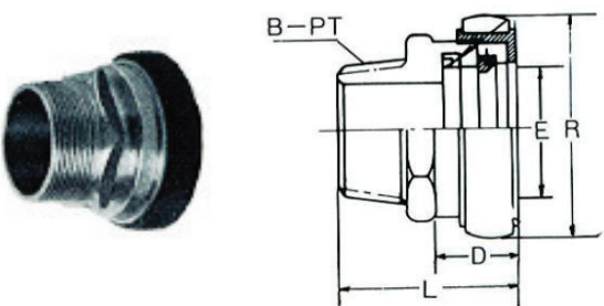
町野式シーベル MBF
