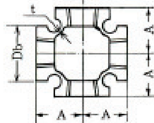
青銅製縁付型(BC-6)
