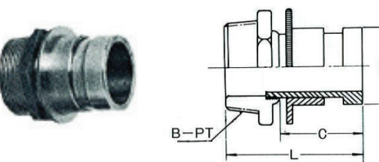
町野式シーベル MBF
