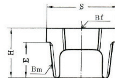
青銅製(BC-6)
