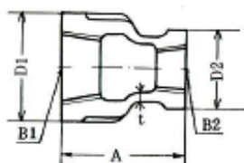
青銅製縁付型 (BC-6)
