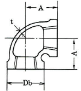
青銅 鑄造縁付型(BC-6)
