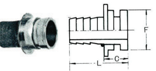
町野式甲型 MBM
