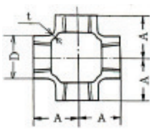
黄銅製平型(C3771)
