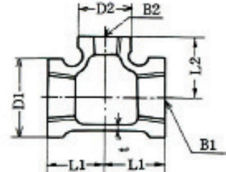
青銅製縁付型 (BC-6)
