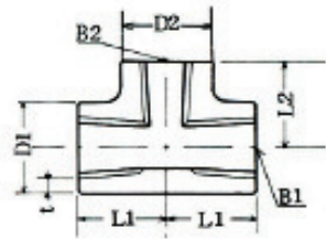
黄銅鍛造製平型(C3771)
