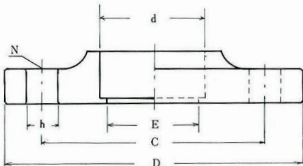
E：適用する銅管の内径
