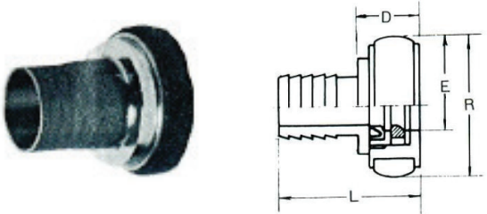
町野式オス MHM
