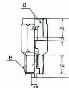
サイフォンパイプ MO MU
