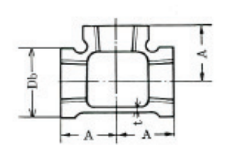
青銅製縁付型 (BC-6)
