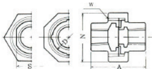
青銅製(BC-6)
