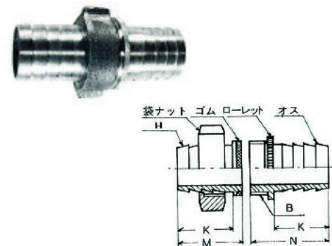
ナミ・ミズグチ WI
