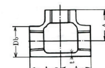
青銅製平型(BC-6)
