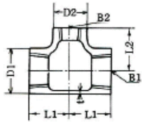
青銅製平型(BC-6)
