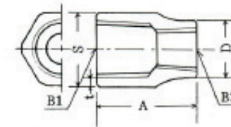
黄銅六角棒製(C3604)
