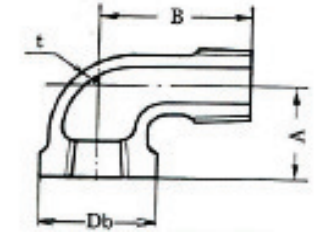
青銅鑄造製縁付型(BC-6)
