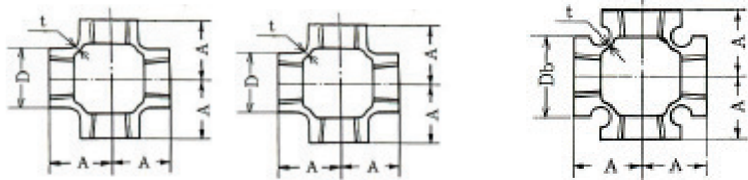
黄銅製平型(C3771)
