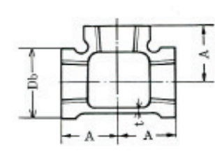
青銅製縁付型(BC-6)
