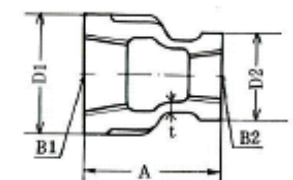
青銅製縁付型(BC-6)
