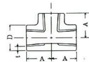
黄銅鍛造製平型(C3771)
