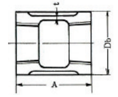
青銅製縁付型(BC-6)
